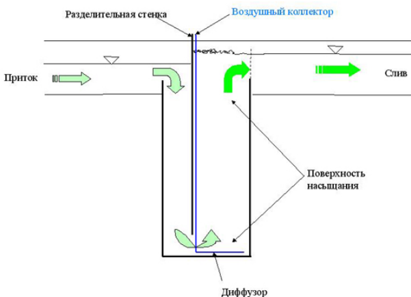
Рис. 5.4. Принцип работы эрлифта
