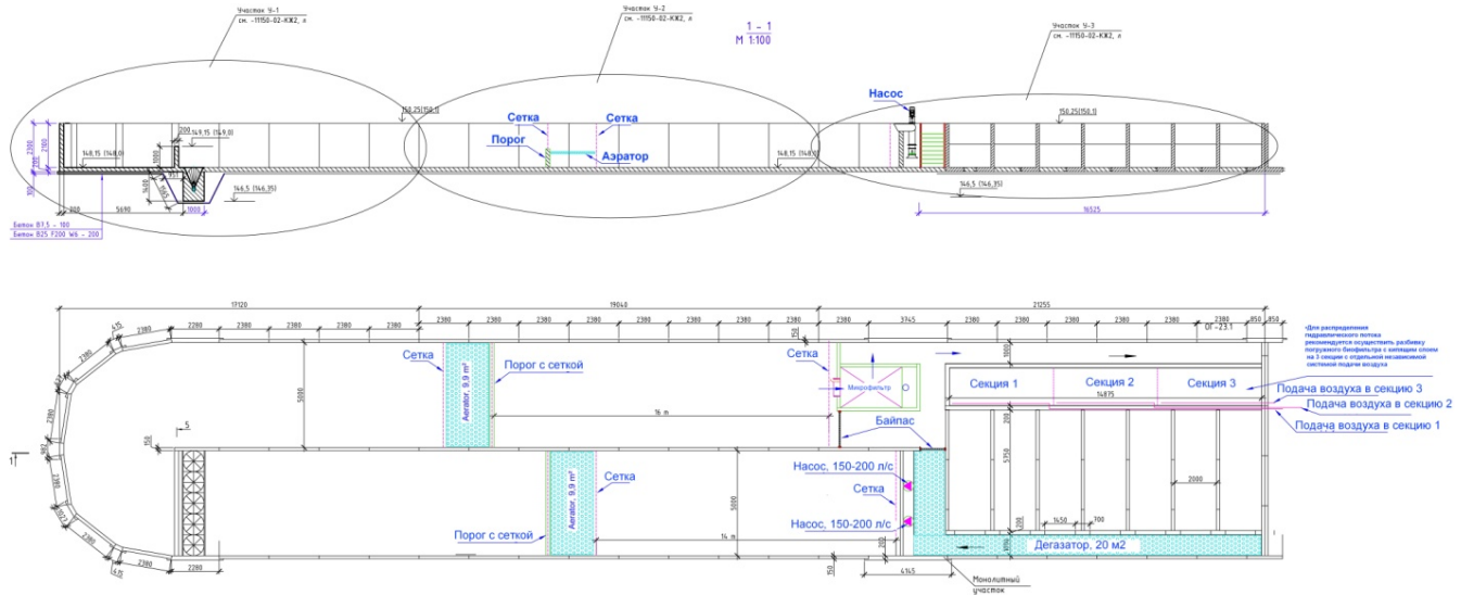
Рис. 1. Предложения по модернизации типовых проектов форелевых УЗВ канального типа
