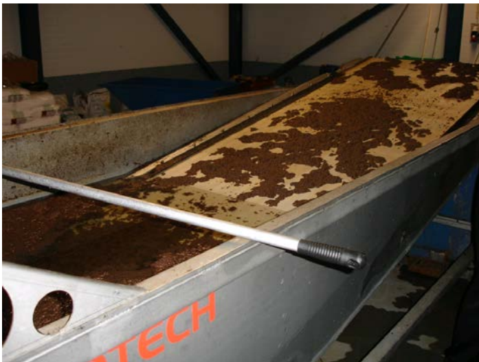
Рис. 5.27. Сепаратор для сточных вод из УЗВ
