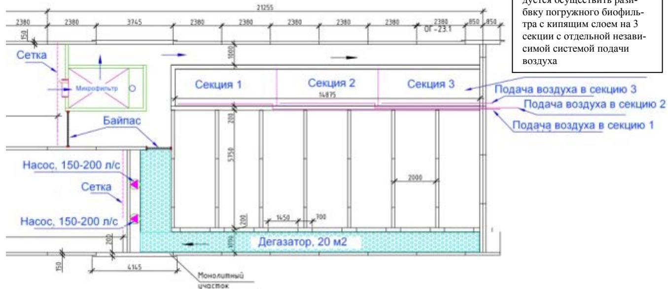
Рис. 2. Предложения по модернизации типовых проектов форелевых УЗВ канального типа (увеличение)
